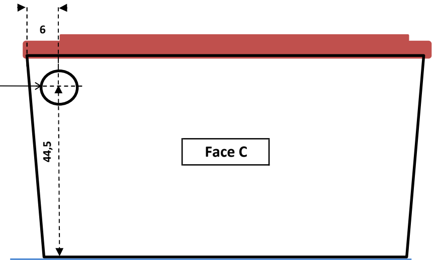
Face C - Sortie des eaux grises pré-filtrées vers coffret
