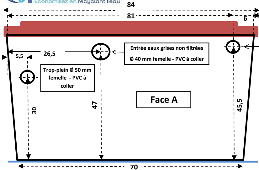
Face A - entrée des eaux grises dans SPAREAU
