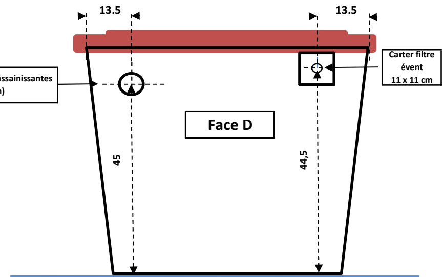
Face D - Côté droit par rapport à la face A
