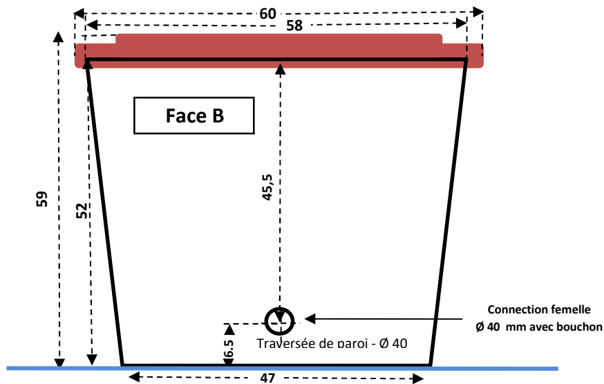
Face B - Côté gauche par rapport à la face A
